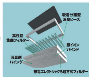
ピュアマリンフィルターの内部構造
